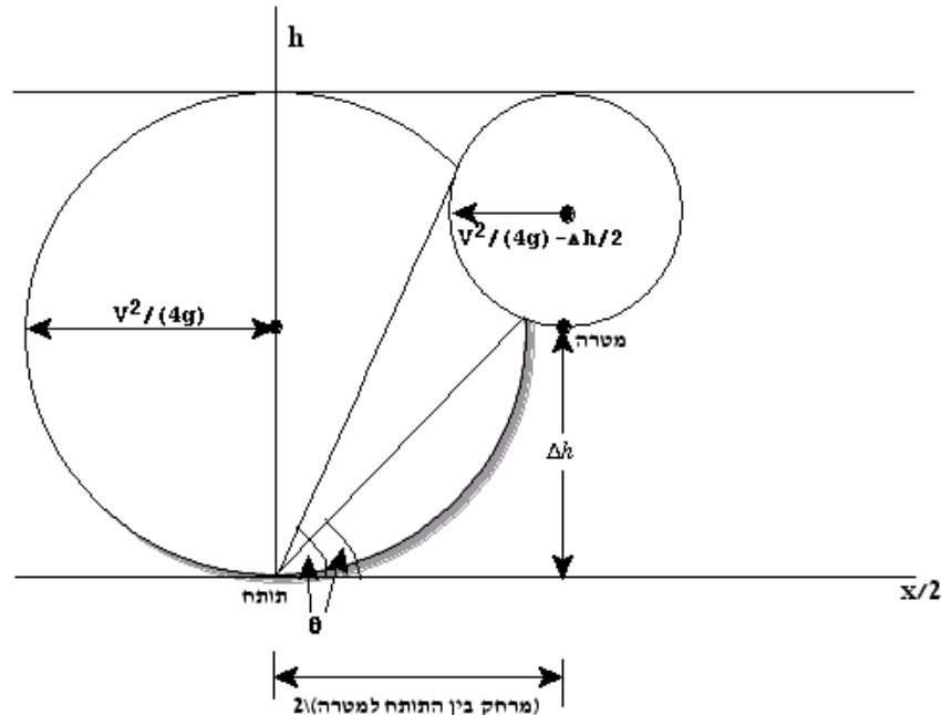
קביעת זווית הירי באופן גרפי עבור תותח ומטרה שונים גובה
